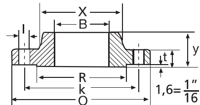
Bridas Slip-On
