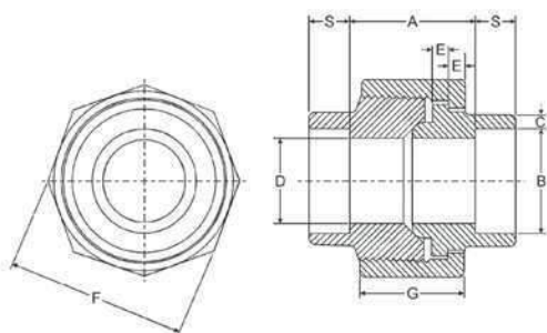
Tuercas unión Socket Welding
