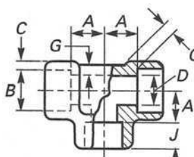
Te
