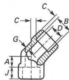
Codo 45°
