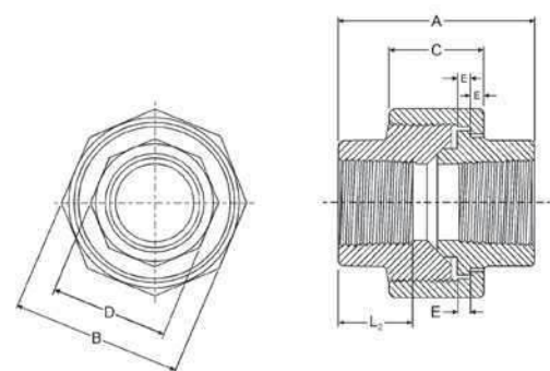
Tuercas unión H-H NPT
